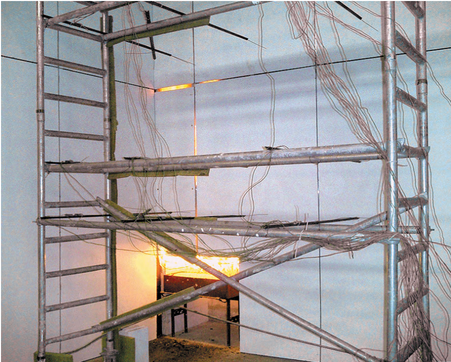
Abb. 8.8: Beginn eines Brandversuchs: Oberhalb der Flamme ist eine hinterlüftete Fassade originalgetreu aufgebaut.
